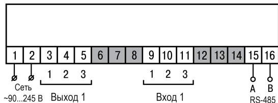
Рисунок 5.2 – Общая схема подключения TRM201-Н, -Щ1 и -Щ2
