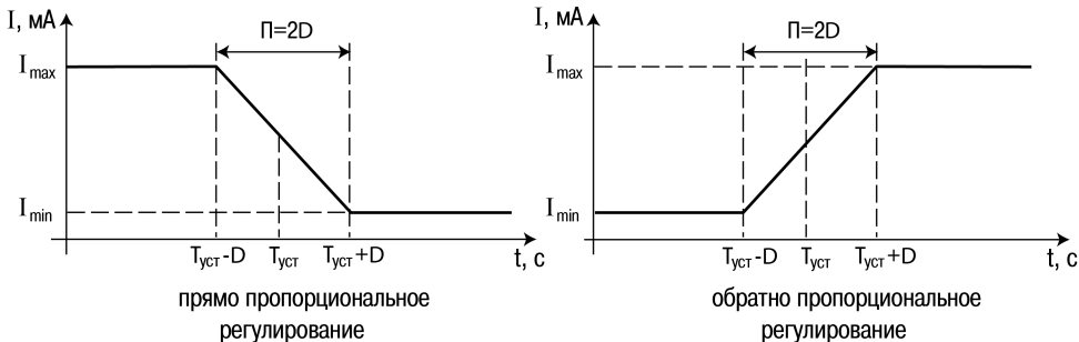
Рисунок 7.8 – Виды регулирования
