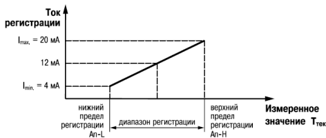
Рисунок 7.6 – Настройка диапазона в случае A_{п.L} < A_{п.H}
