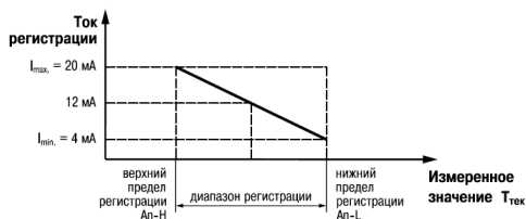
Рисунок 7.7 – Настройка диапазона в случае A_{п.L} > A_{п.H}
