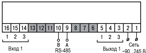
Рисунок 5.3 – Общая схема подключения TRM201-Н2
